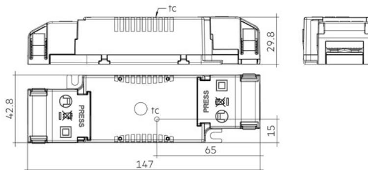
Maßskizze
