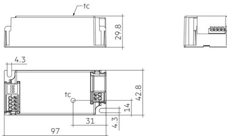
Maßskizze
