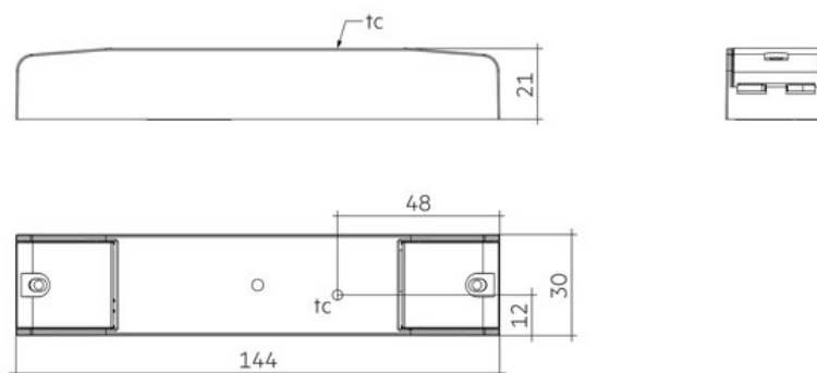
Maßskizze
