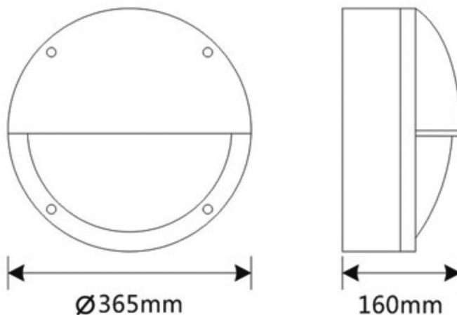
Maßskizze
