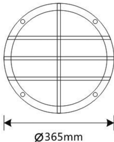
Maßskizze
