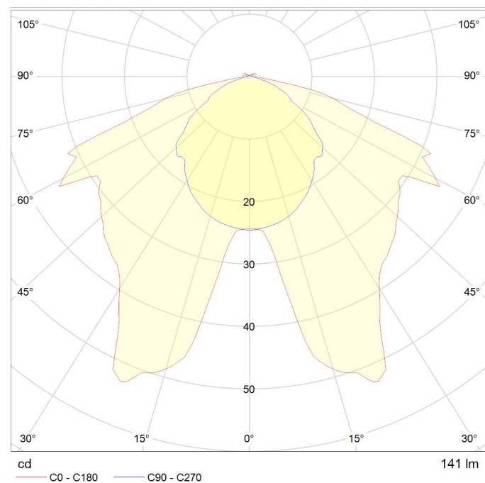
Lichtverteilungskurve
