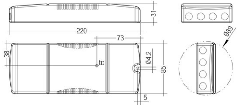
Maßskizze
