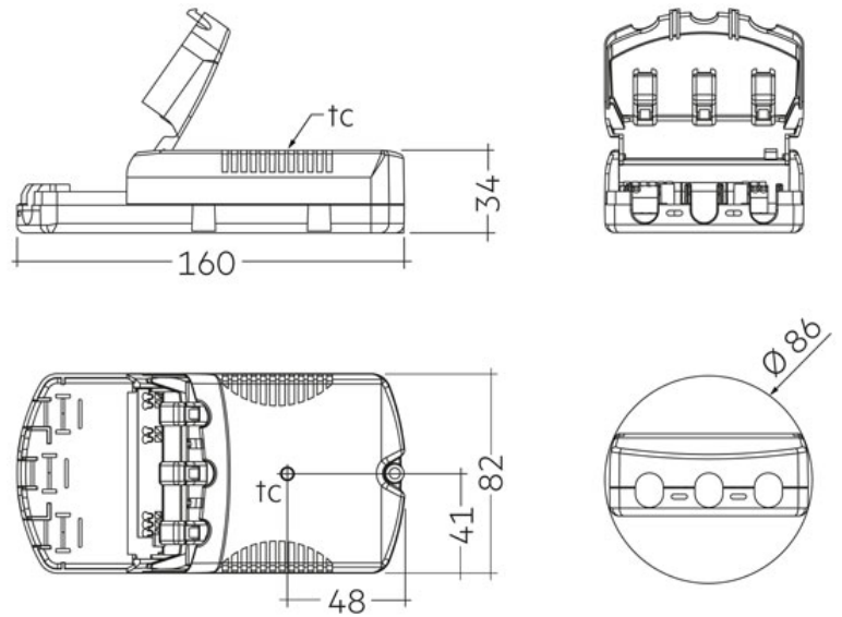
Maßskizze
