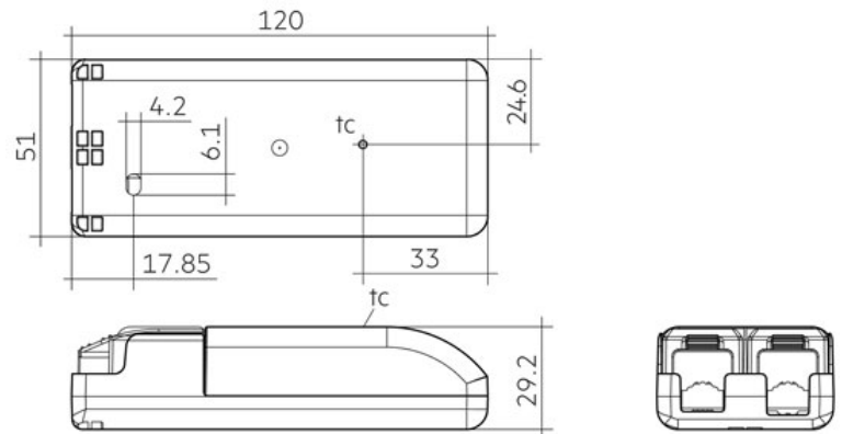
Maßskizze
