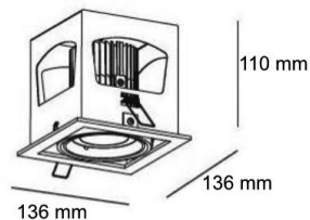
Deckenausschnitt: 120 mm x 120 mm
